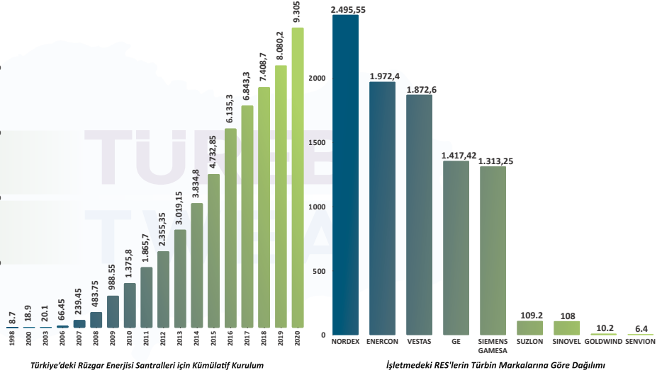
Türkiye'deki Rüzgar Enerjisi Santralleri için Kümülatif Kurulum
