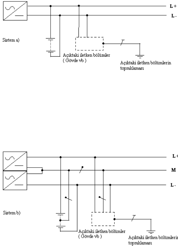
Şekil-5j TT Doğru akım sistemi
