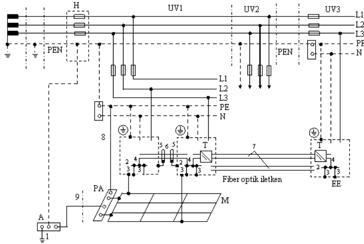
Şekil-28 Aynı şebeke beslemesinin başka bir alt dağıtım panosundan beslenen ve ekransız, galvanik olarak ayrılmış sinyal iletim hatlarıyla bağlanan uzaktaki bir son cihaza sahip iletişim tesisinin topraklamasına örnek (Not: Bu şekil mecburi olmayıp, yalnızca bir fikir vermek amacıyla taşınmaktadır.)
