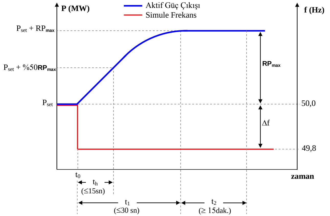
Şekil E.17.A.4 - f=49,8 Hz'lik Simule Frekans Uygulamasında Üniteden Beklenen Tepki
